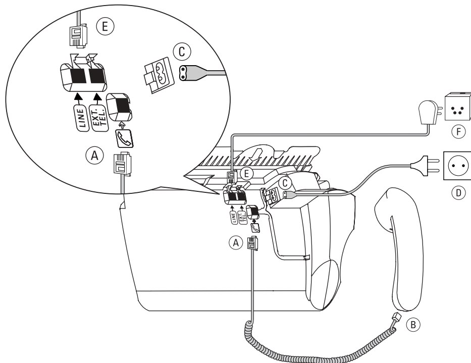
Afbeelding 1: Pacific 100 aansluiten.
